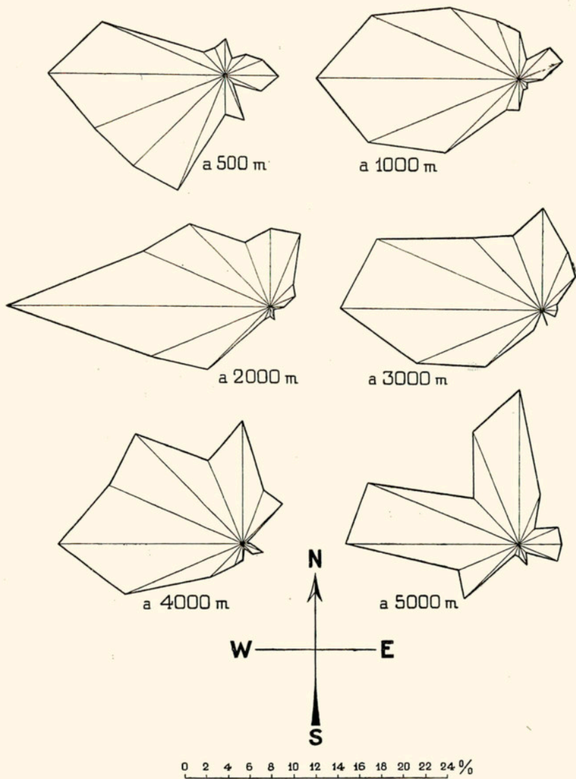
Fig. 1. — Freqüència, en tant per cent del total d'observacions, de les direccions del vent a Barcelona, a diverses altituds, durant l'any 1931
