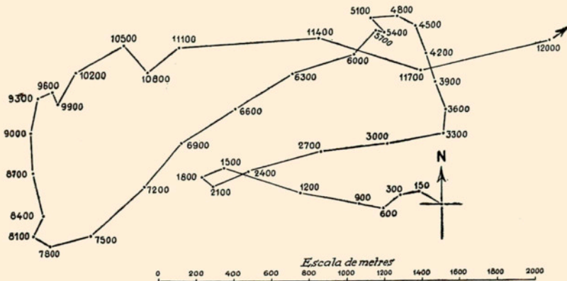
Fig. 3. — Trajectòria del globus del 2 de novembre de 1931, a les 11 h 45 m . (Règim anticiclònic amb poc vent.)
